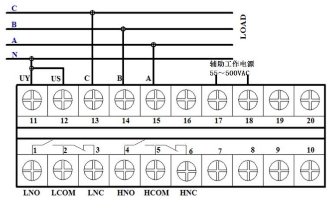
三相四线制接线
